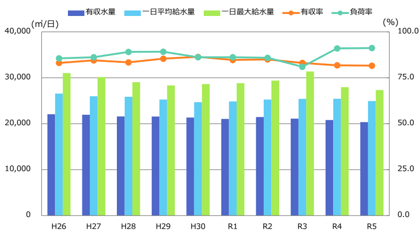
図 5-2 水需要の実績
