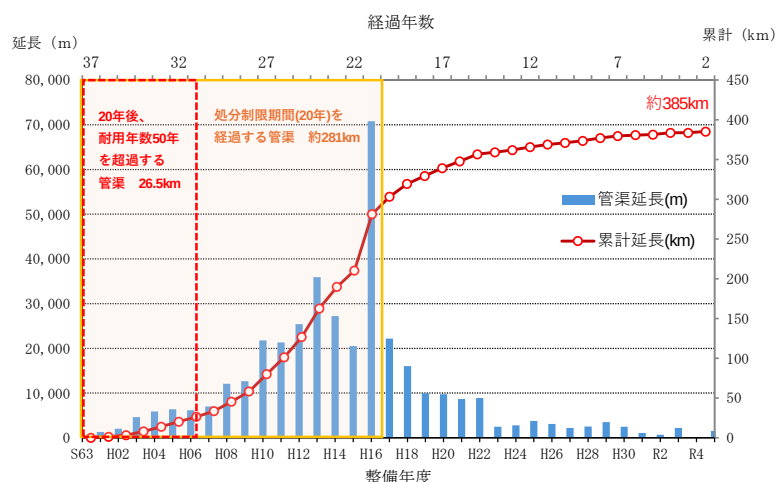
図 6-5 整備年度別管渠延長（下水道事業 R5 末時点）
