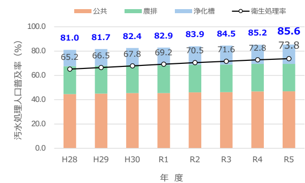
図 6-1 汚水処理人口普及率等の推移
