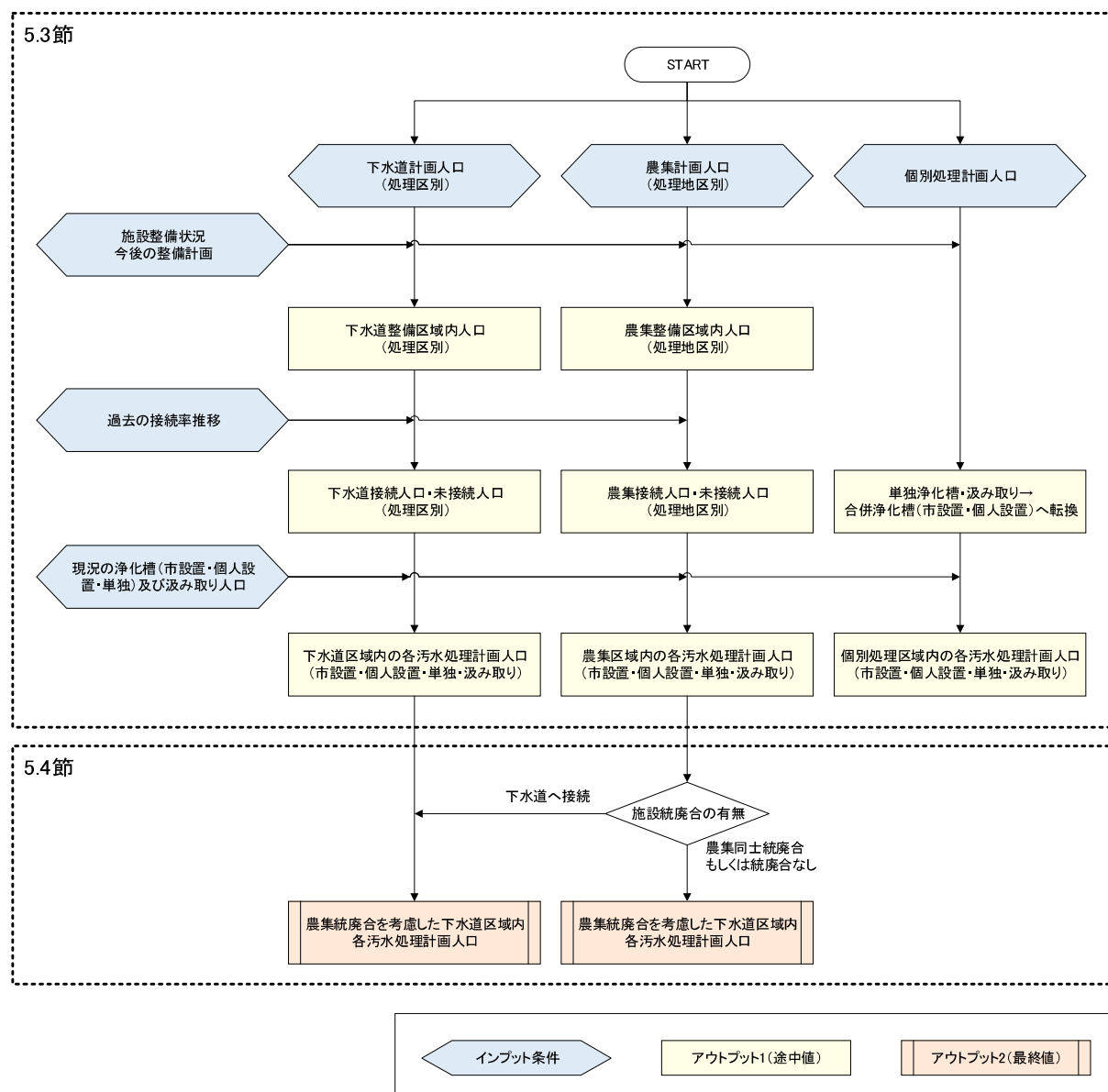
図 5-7 本節及び次節における年度別計画人口の検討フロー
