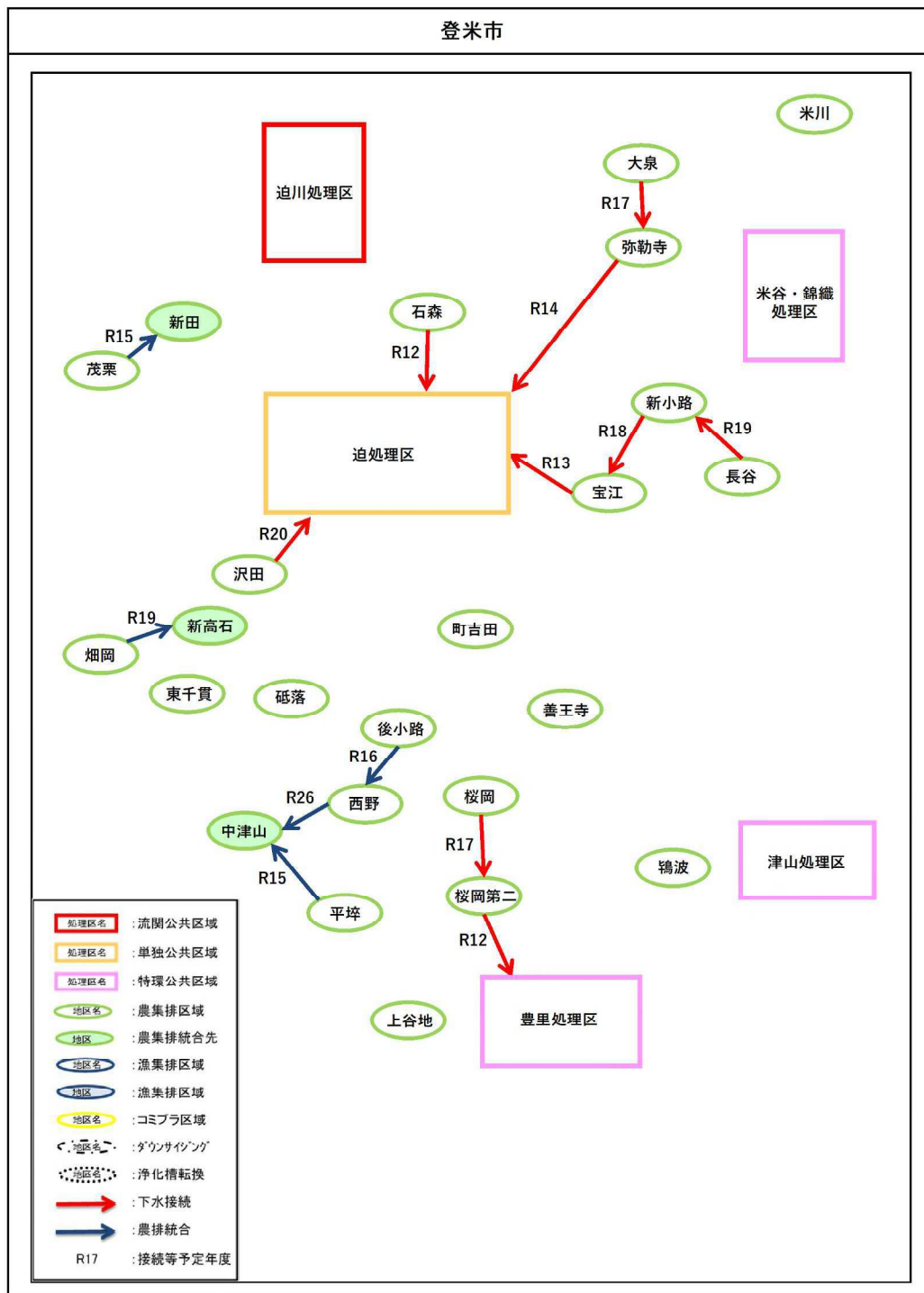
図 5-14 施設統廃合計画の概要（宮城県様式 5）
